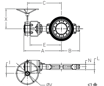
EN 1092-1 PN 10 / PN 16 - Trim B
